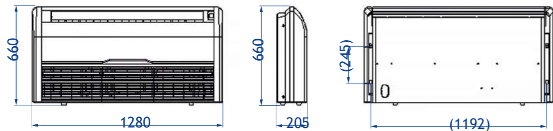
ALCF-H30NDR3HA, ALCF-H36NDR3HA, ALCF-H42NDR3HA ALCF-H48NDR3HA, ALCF-H60NDR3HA
