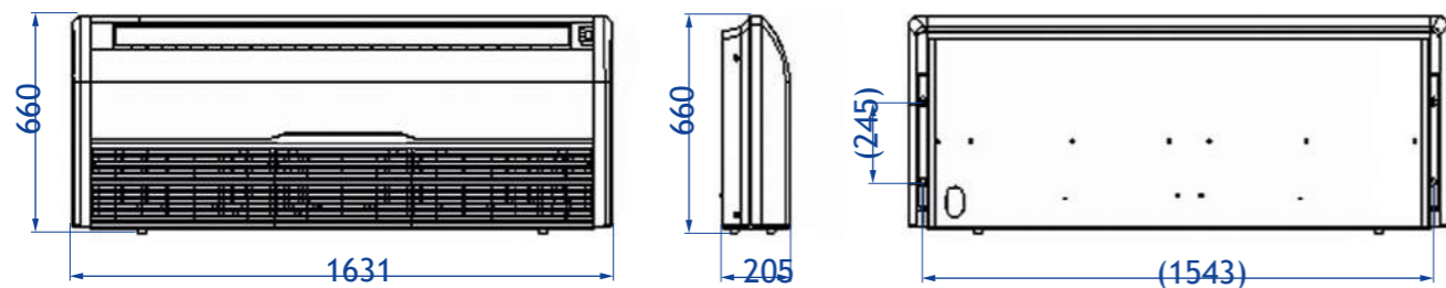
ALCF-H30NDR3HA, ALCF-H36NDR3HA, ALCF-H42NDR3HA ALCF-H48NDR3HA, ALCF-H60NDR3HA
